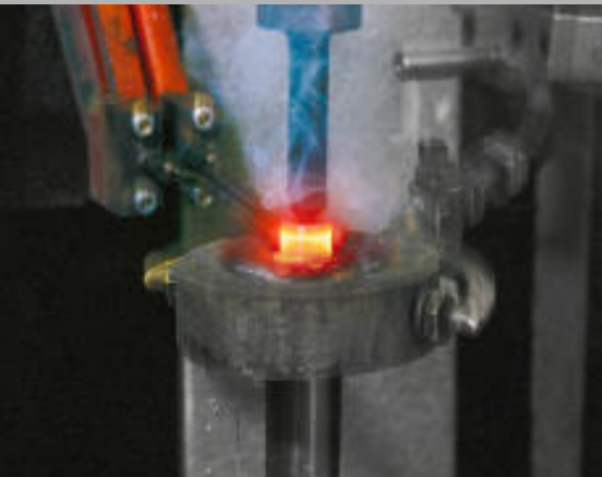
Durcissement inductif
