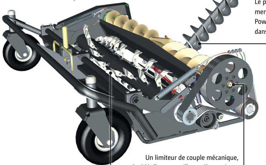
Unité de tonte frontale SmartCut
